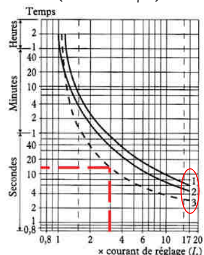
Courbe de déclenchement LR2-D Classe 20 A (Télemécanique)
